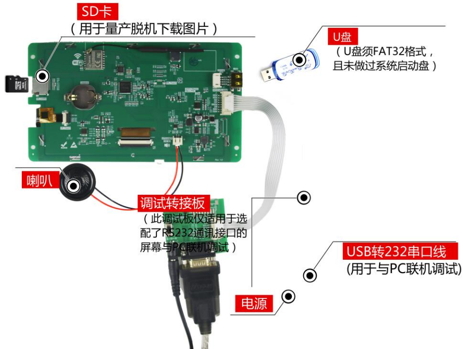
图 1-5 调试工具图
