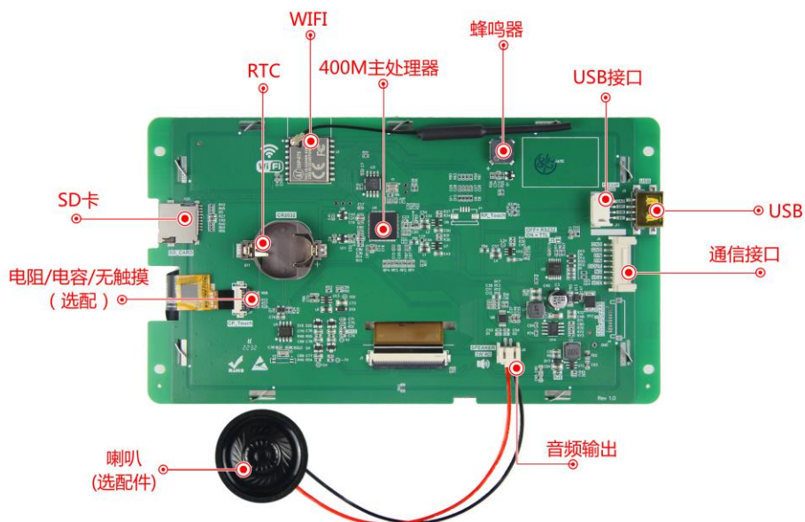
图 1-4 硬件配置图
